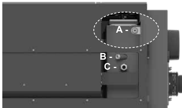
Hülseposition für Abgasfühler - TSV (A), Kesseltemperaturfühler - TK (B) und Pumpenthermostat (Mutterart) für die Pumpe TČ 70 °C (C)
